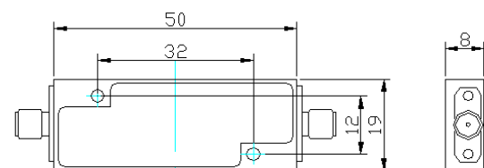
俯视图
