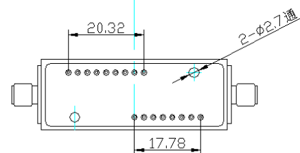
底视图
